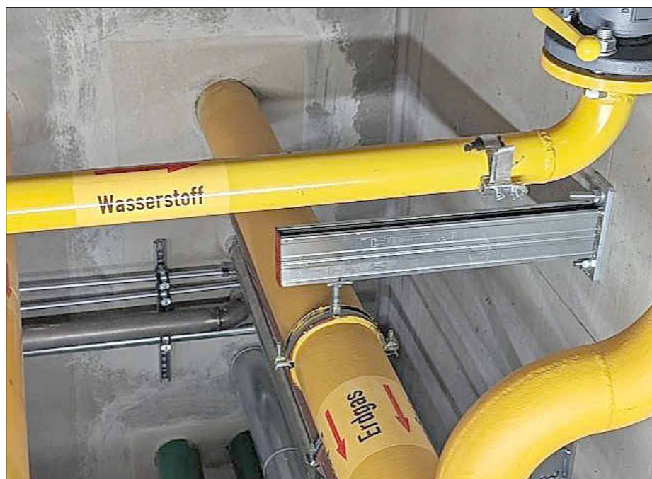
In der Wasserstoffproduktionsanlage Wunsiedel, Foto: Jürgen Reinwald
